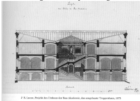
Lucae: Bauakademiequerschnitt
