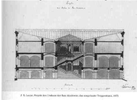
Lucae: Bauakademiequerschnitt
