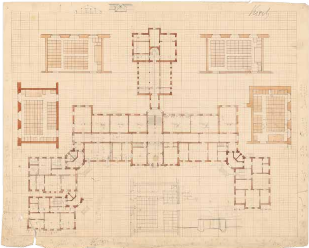
Abbildung 2 Gustav Knoblauch: Lehrerseminar Kyritz, Grundrißstudie, um 1871
