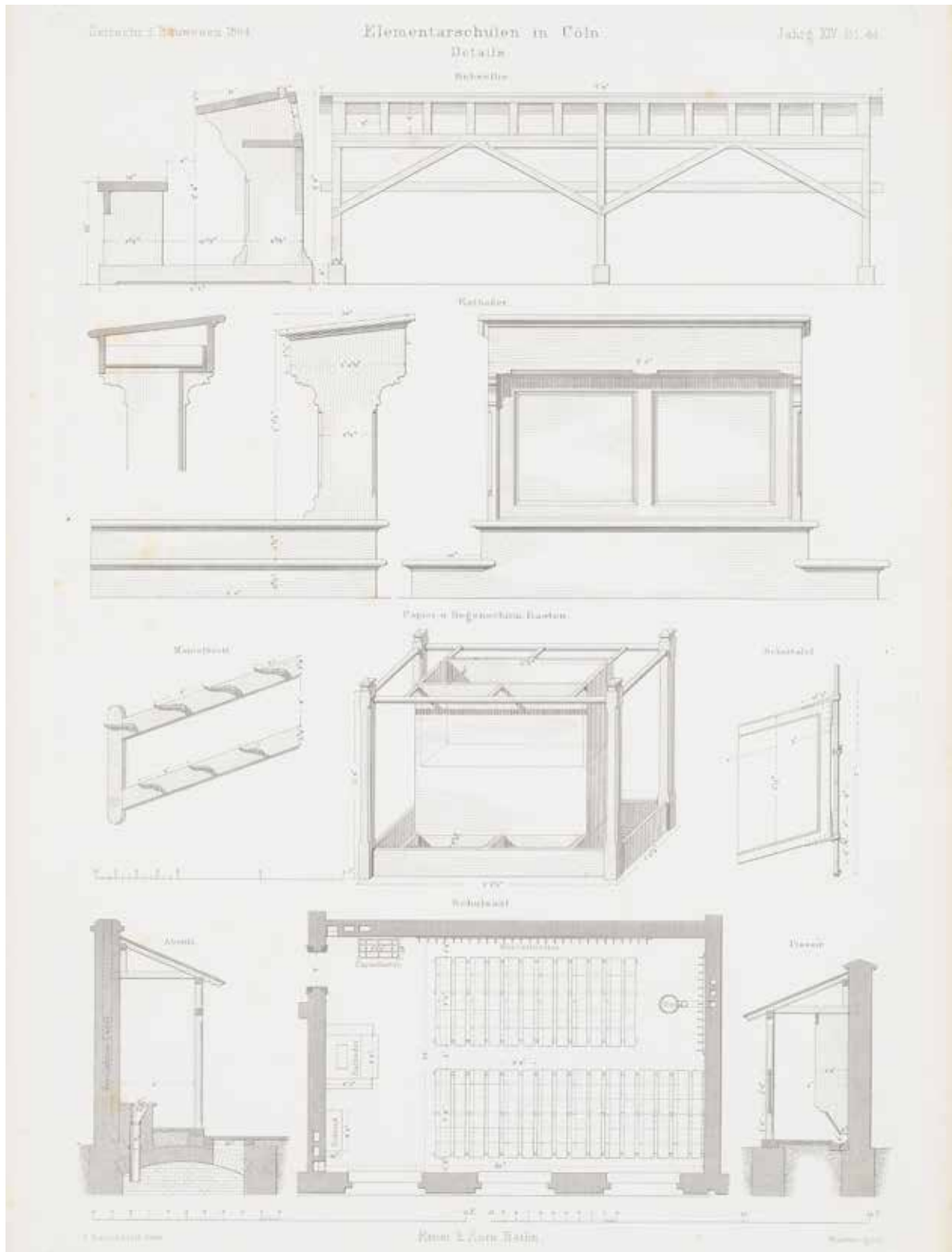
Abbildung 1 Entwurf für das Mobiliar und die Toiletten der Elementarschulen Köln. Stich aus der Zeitschrift für Bauwesen, 1864
